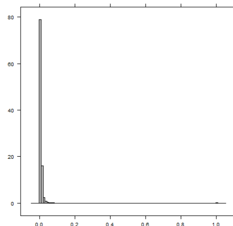
Figure A5 : Histogramme de la mesure de l'ASM (Angular Second Moment) de r.texture (échelle des ordonnées x 10000)
