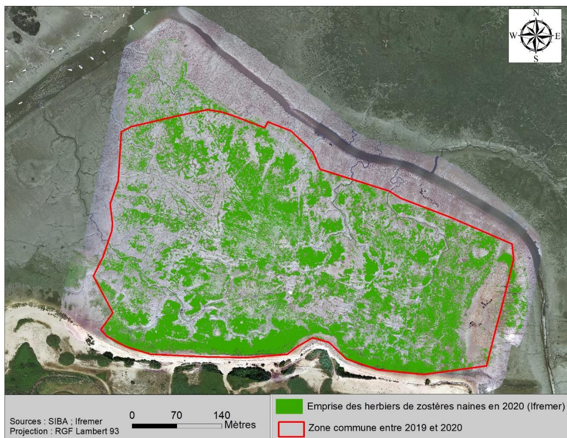
Figure 8 : Carte de l'emprise des herbiers de Zostera noltei à l'été 2020 obtenu par classification d'image supervisée.
