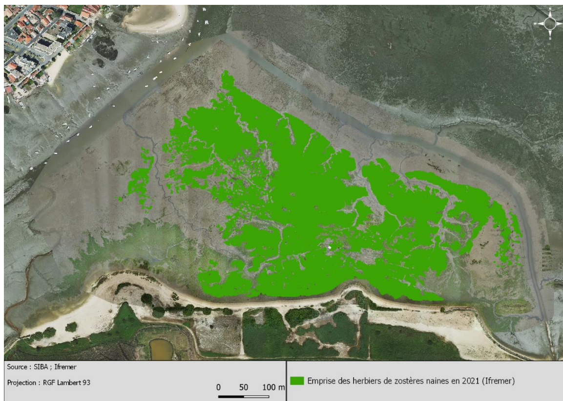
Figure 9 : Carte de l'emprise des herbiers de Zostera noltei à l'été 2021 obtenue par numérisation de l'ortho mosaïque géoréférencée.
