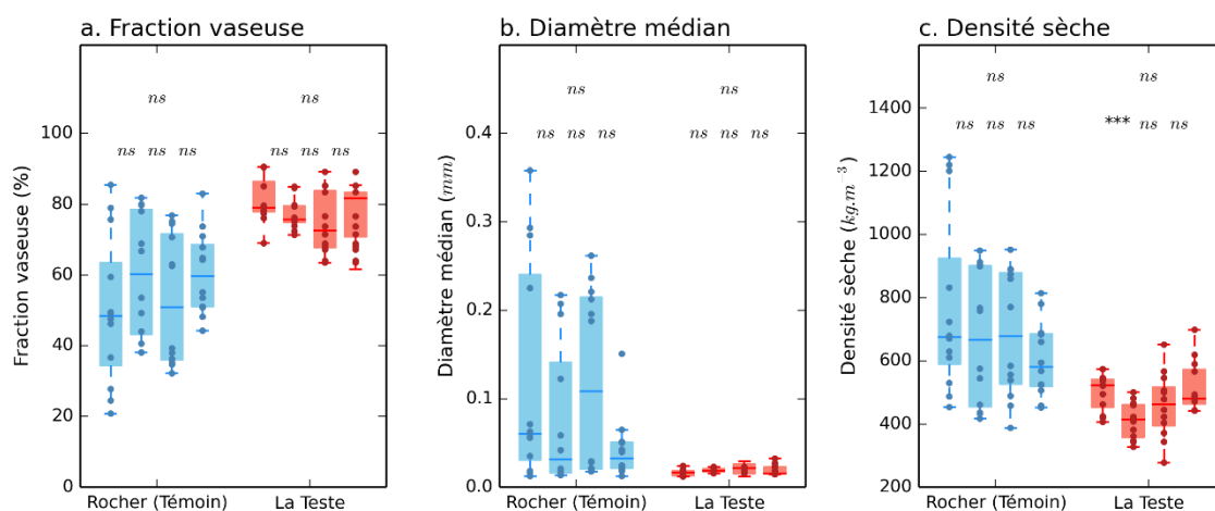
Figure 24 : Comparaison des caractéristiques des sédiments superficiels avant travaux, entre 2019 et 2022 pour les grilles Rocher (référence en bleu) et La Teste (en rouge), pour (a) la fraction vaseuse, (b) le diamètre médian et (c) la densité sèche.
