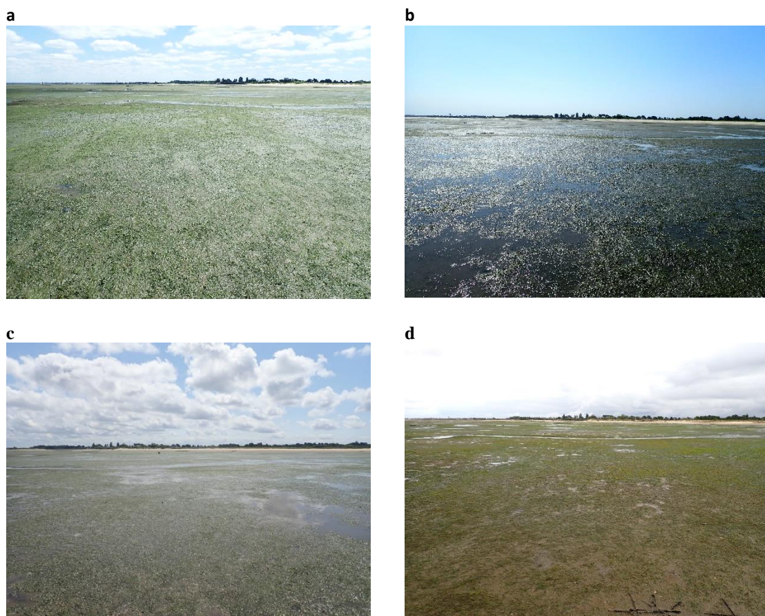
Figure 15 : Vue générale de la station de référence « Rocher Témoin » (a) en 2019, (b) en 2020, (c) en 2021 et (d) en 2022.
