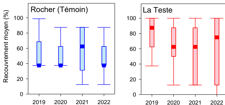
Figure 21 : Boîtes à moustaches 3 présentant le recouvrement des zostères (%) sur les deux grilles au cours des quatre années.
