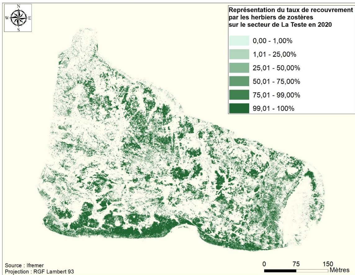
Figure A11 : Représentation du taux de recouvrement par les herbiers de zostères naines sur le secteur de La Teste en 2020.
