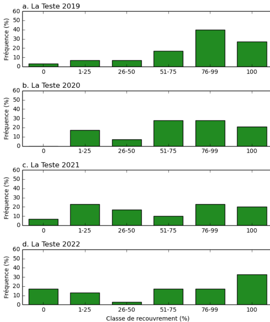
Figure 20 : Distribution du recouvrement des zostères sur les 30 points de la station « La Teste » (a) en 2019, (b) en 2020, (c) en 2021 et (d) en 2022.
