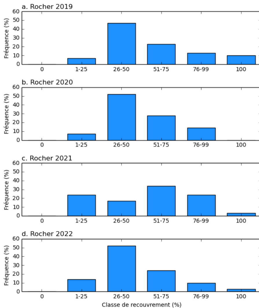
Figure 17 : Distribution du recouvrement des zostères sur les 30 points de la station « Rocher Témoin » (a) en 2019, (b) en 2020, (c) en 2021 et (d) en 2022.
