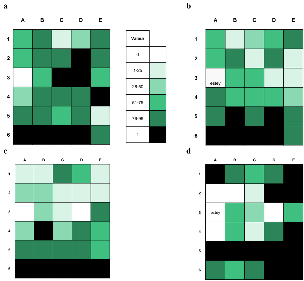
Figure 19 : Taux de recouvrement des zostères sur les 30 points de la station « La Teste » (a) en 2019, (b) en 2020, (c) en 2021 et (d) en 2022.
