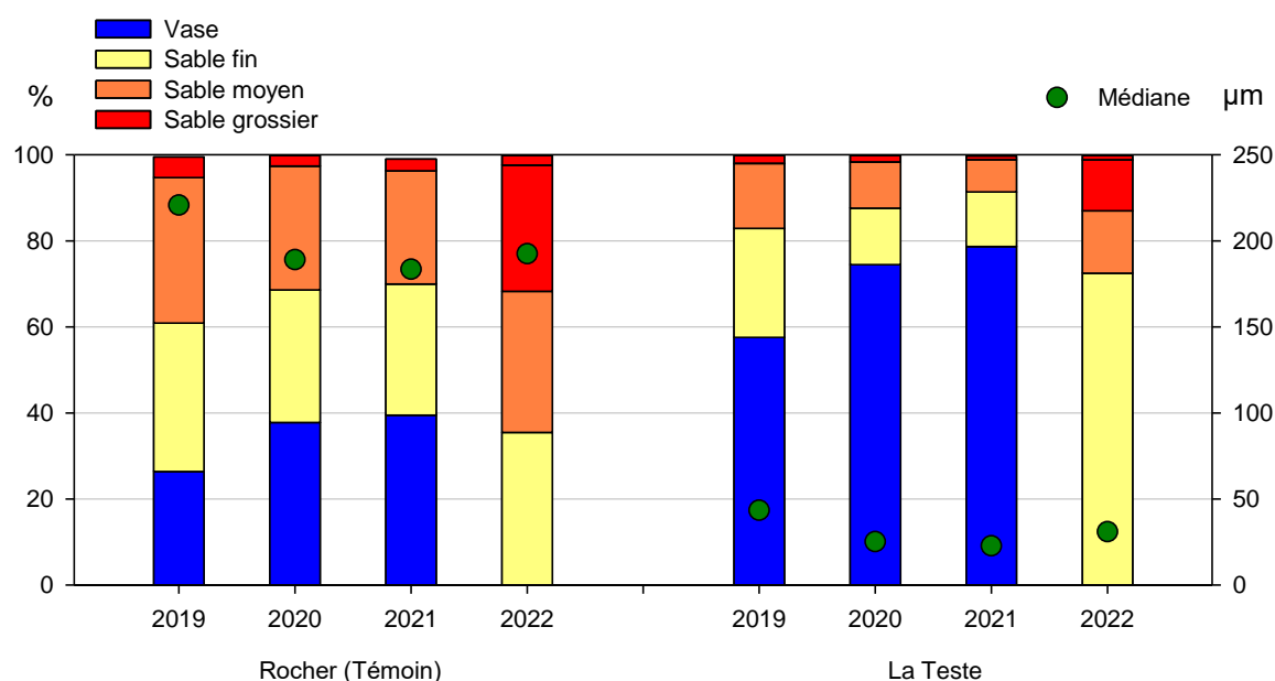
Figure 23 : Caractérisation granulométrique des sédiments des deux grilles suivies.
