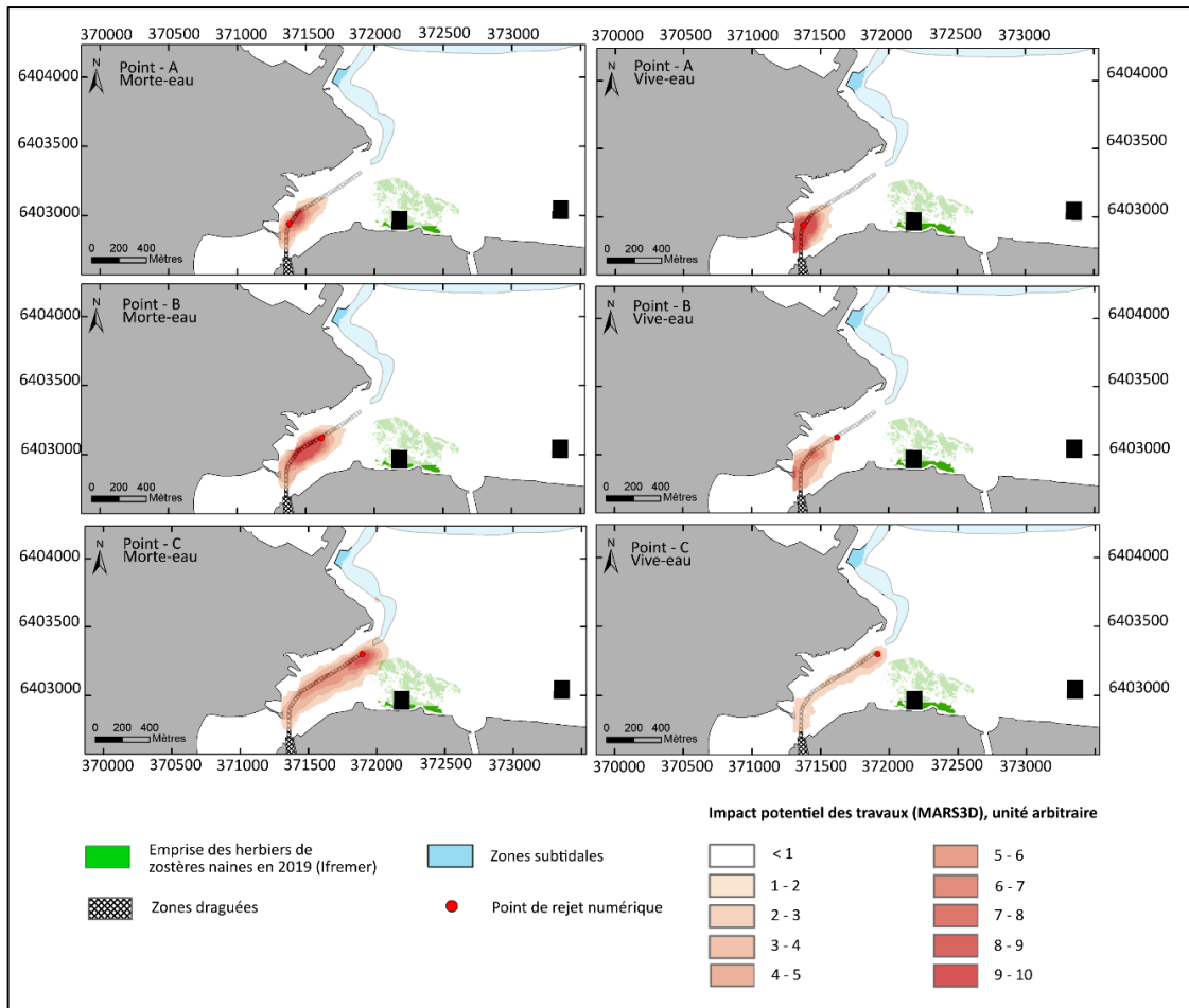
Figure 4 : Résultats détaillés de la modélisation de l'impact des travaux dans le secteur de La Teste de Buch.
