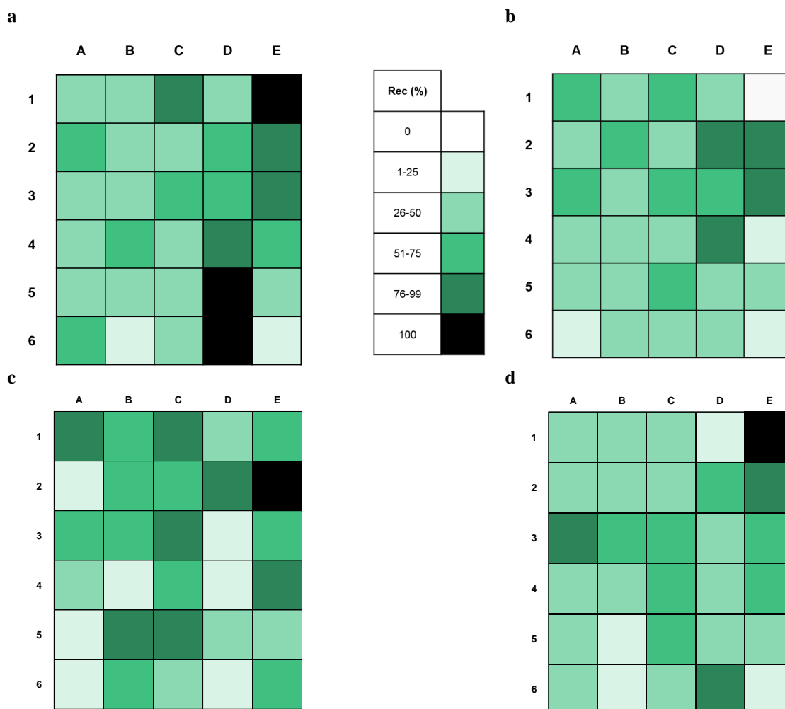
Figure 16 : Taux de recouvrement des zostères sur les 30 points de la station « Rocher Témoin » (a) en 2019, (b) en 2020, (c) en 2021 et (d) en 2022.
