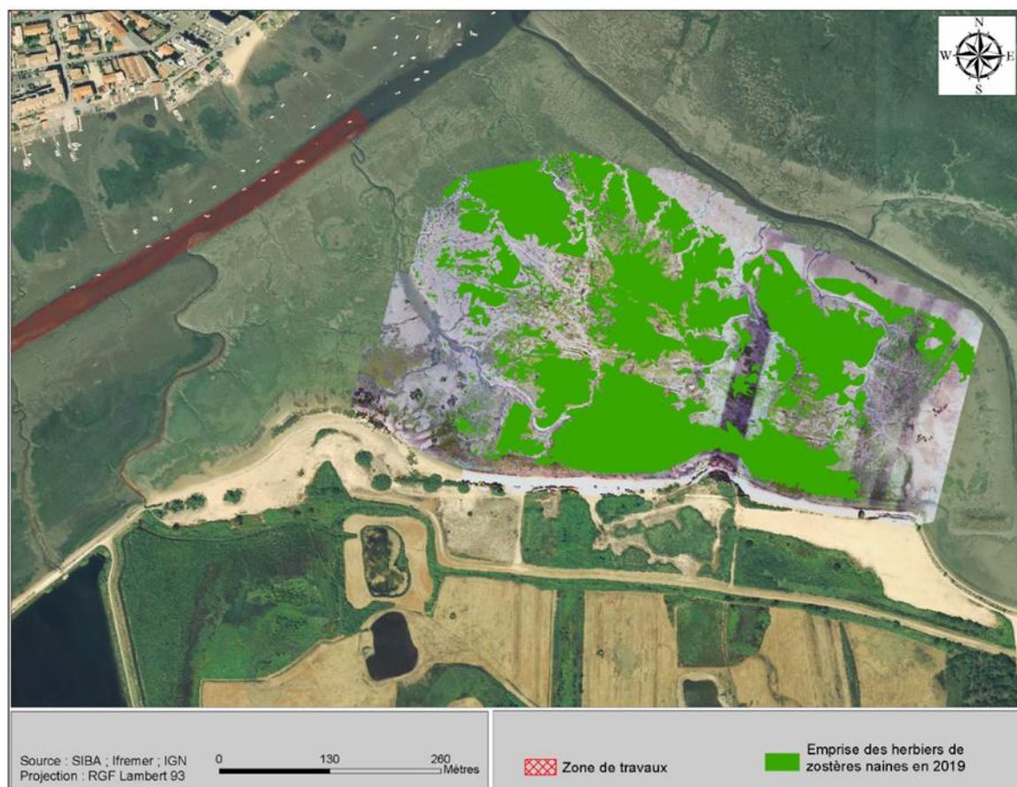
Figure 6 : Carte de l'emprise des herbiers de Zostera noltei à l'automne 2019 obtenue par numérisation de l'ortho mosaïque géoréférencée.
