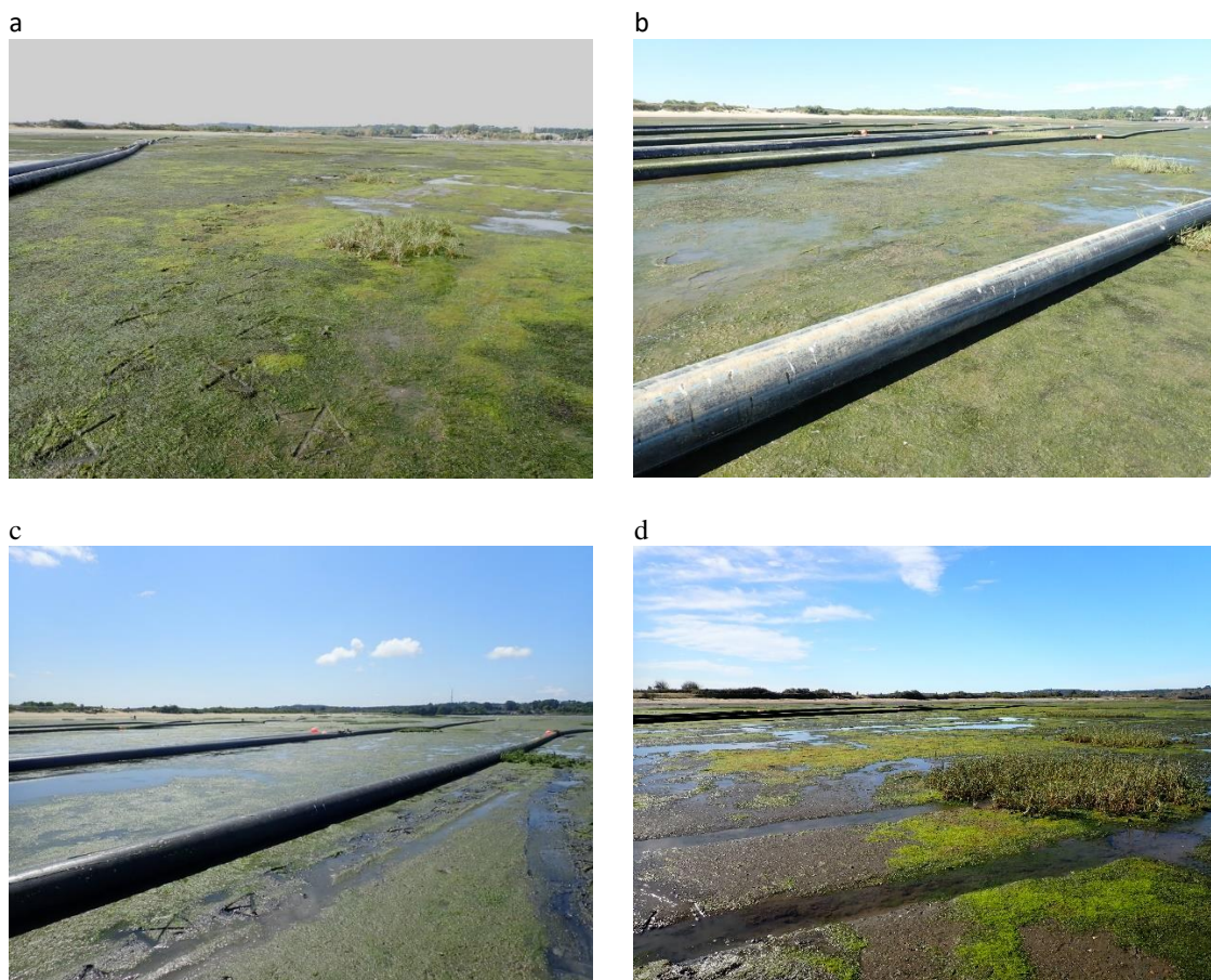
Figure 18 : Vue générale de la station « La Teste » (a) en 2019, (b) en 2020, (c) en 2021 et (d) en 2022.
